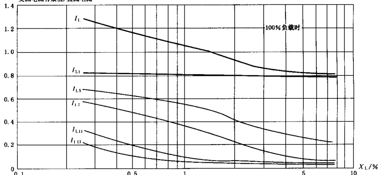
图 B. 9 输入谐波电流
