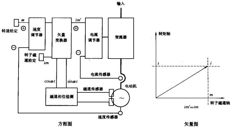
图 D.6 带磁通检测的磁通定向控制(电压源型变频器)
