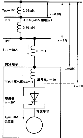
图 B.11 简单结构举例
