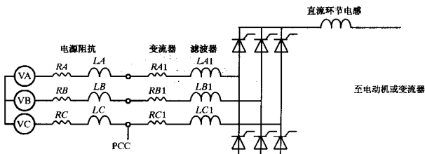
图 B.1 具有大直流电感的晶闸管变流器
