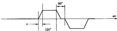
图 B.3 梯形波线电流
