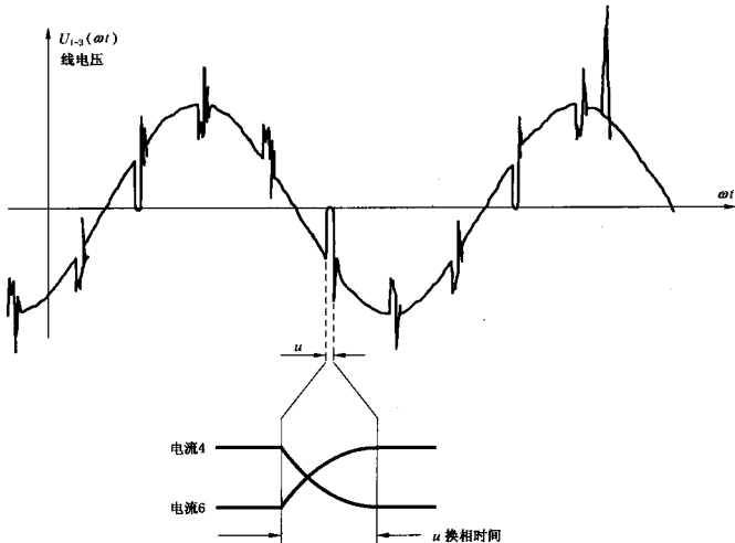
图 B.13 3相6脉波桥式变流器的换相缺口
