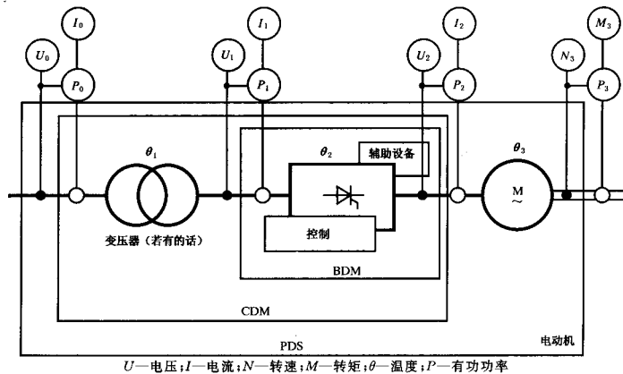
图8 PDS的测试电路
