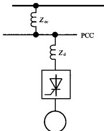
图 B.14 用于评估换相缺口减小的等效电路
