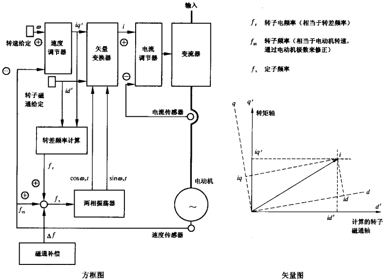
图 D.7 带转差频率计算的磁通定向控制(电压源型变频器)
