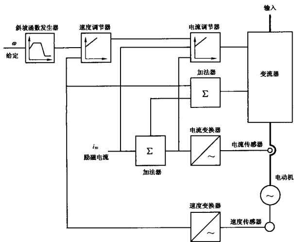
图 D.5 直接转速控制(电压源型变频器)
