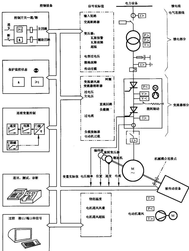
图 1 交流传动系统功能方框图
