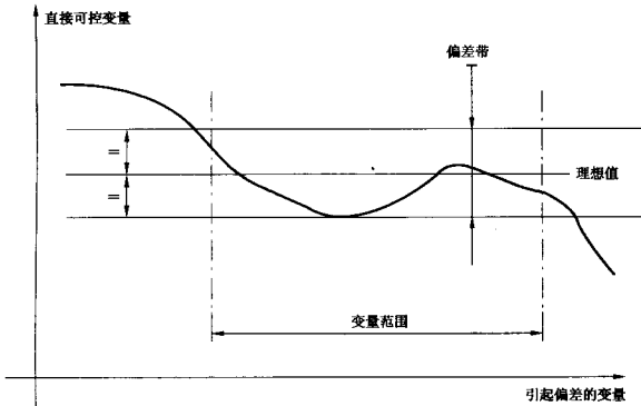
图 7 偏差带
