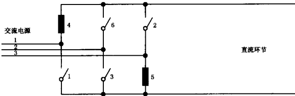
图 B.12 3相6脉波桥式变流器
