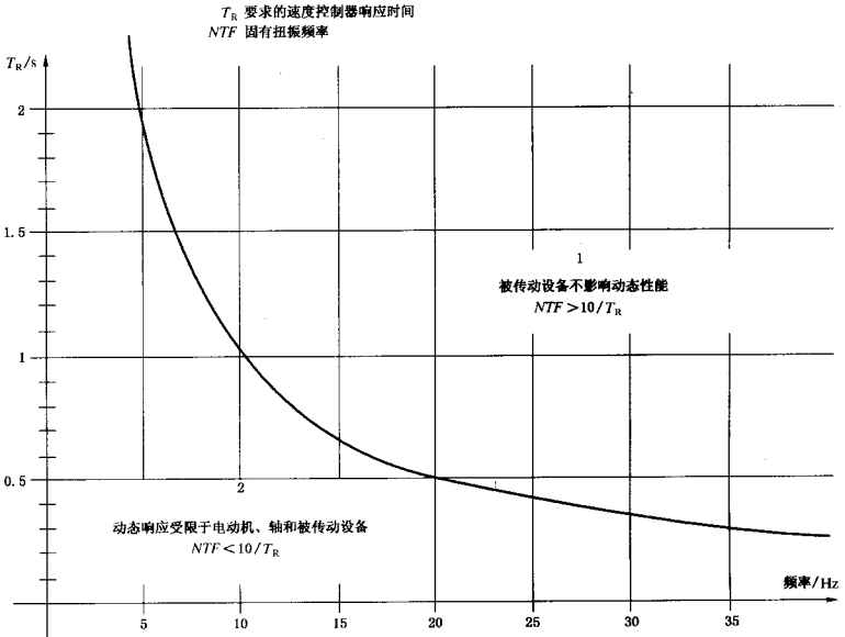
图 D.14 简单的扭振稳定性准则
