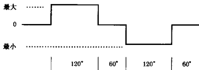
图 4 准矩形波
