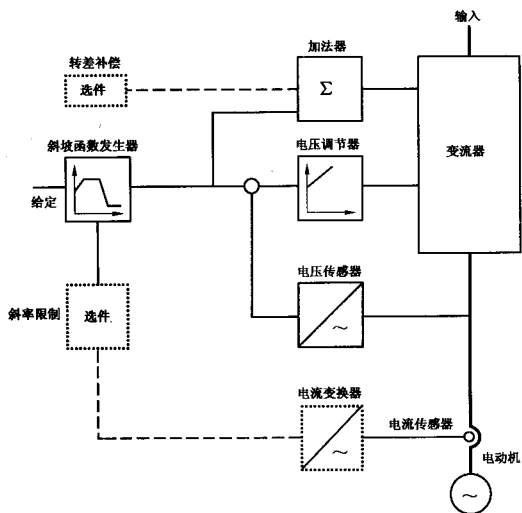
图 D.4 V/F 控制(电压源型变频器)
