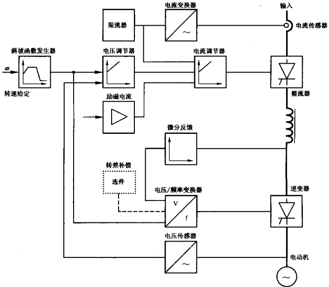
图 D.2 V/F 控制(电流源型变频器)
