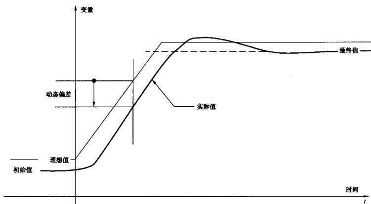
图 D.10 随给定以规定的速率变化的时间响应
