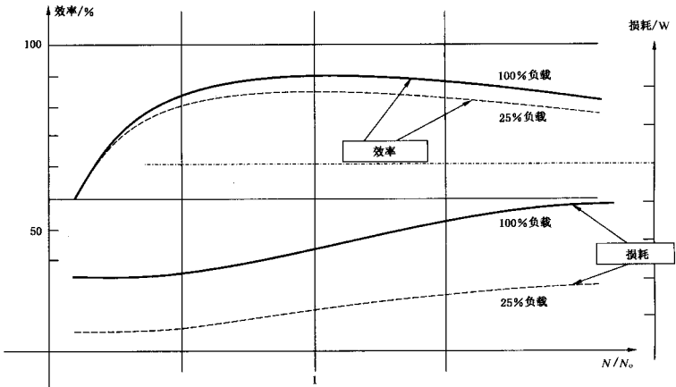
图 6 PDS 效率和损耗的典型曲线
