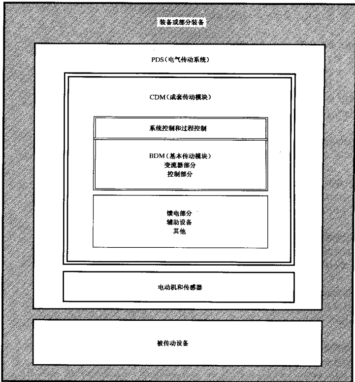
图 2 装备内 PDS 的硬件配置
