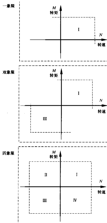
图 3 运行象限
