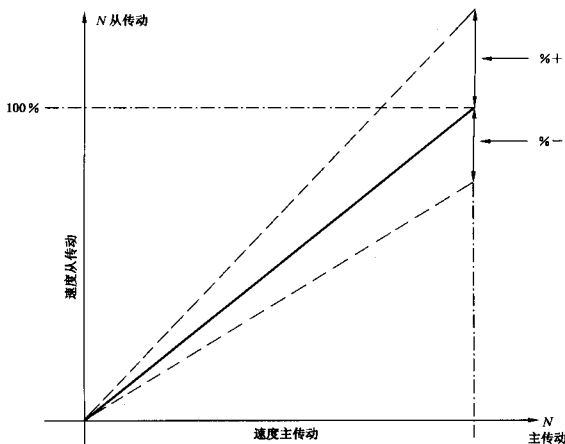
图 D.11 主/从传动系统
