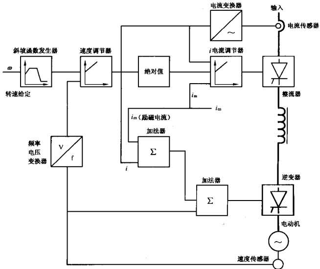
图 D.3 直接转速控制(电流源型变频器)
