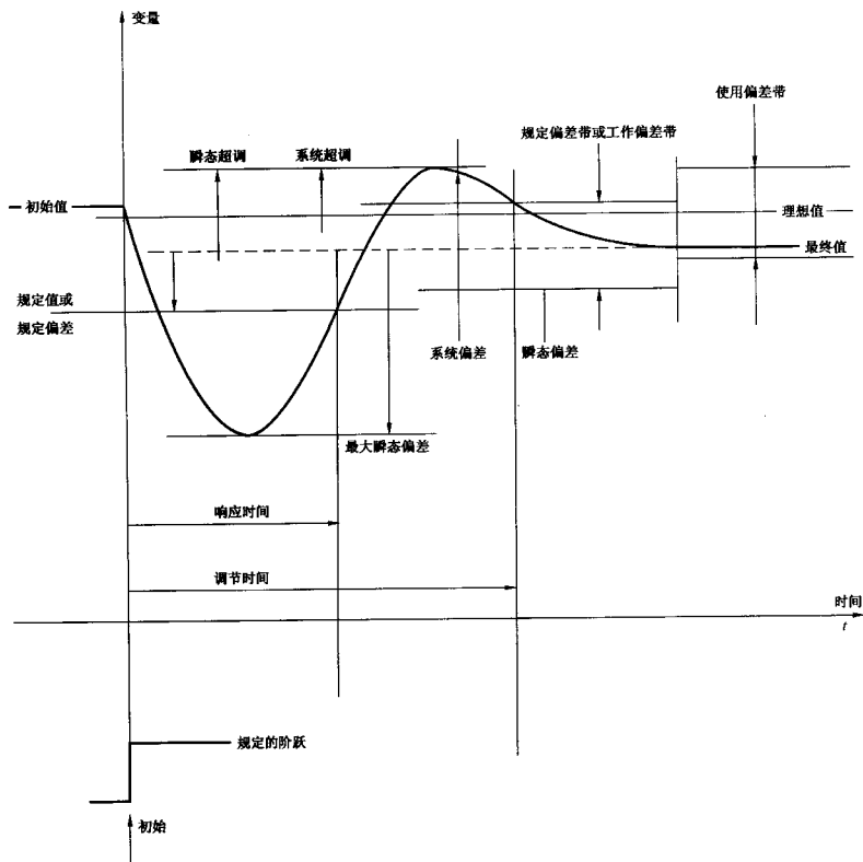
图 D.9 随负载阶跃增加的时间响应——给定不变
