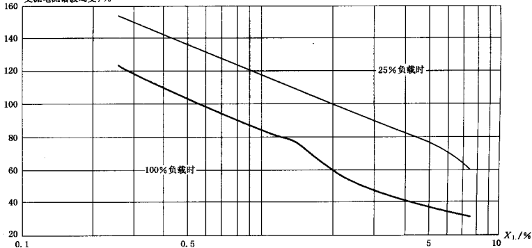
图 B. 10 输入电流畸变
