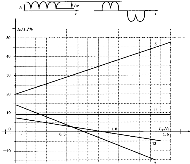
图 B.4 电源电流的主要谐波分量,假定方波线电流具有理想的直流电流纹波
